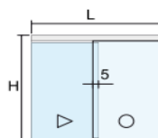
INSTALACIÓN RIEL CON CANAL PARA FIJO
