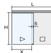
INSTALACIÓN RIEL SENCILLO A MURO
